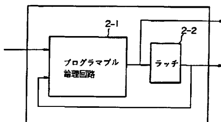
プログラマブル論理セルの構成
